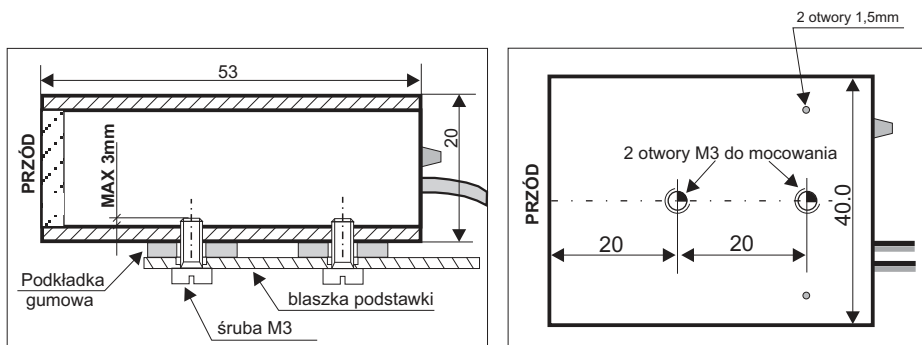
Rysunek obudowy woltomierza "od spodu"
