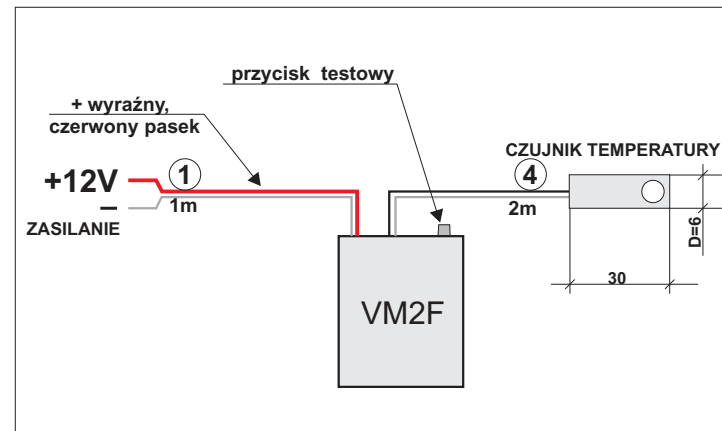
Schemat podłączenia miernika do instalacji elektrycznej.
